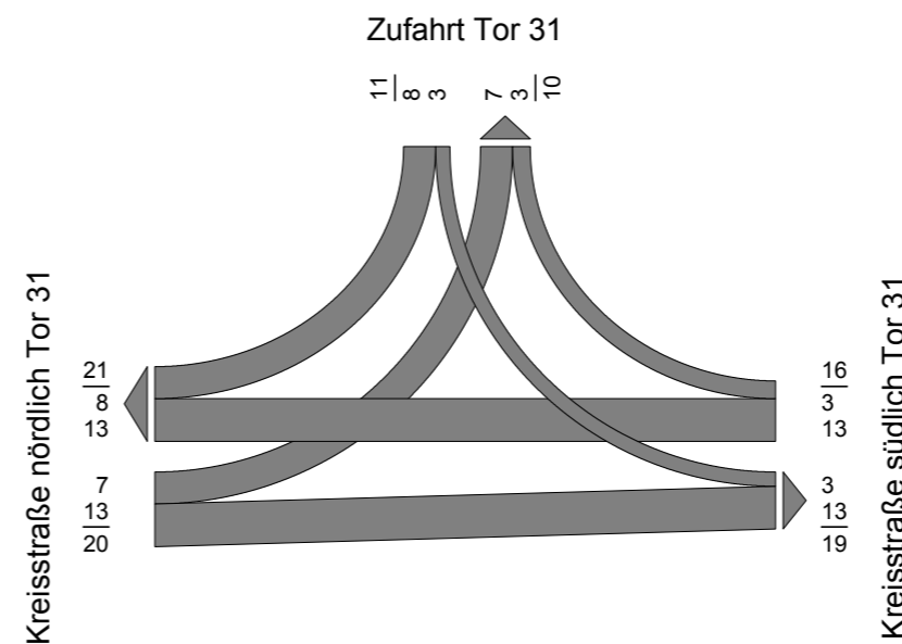
Knotenströme Mittlere Nachtbelastung (22:00 Uhr - 6:00 Uhr) in Lkw/Std.
