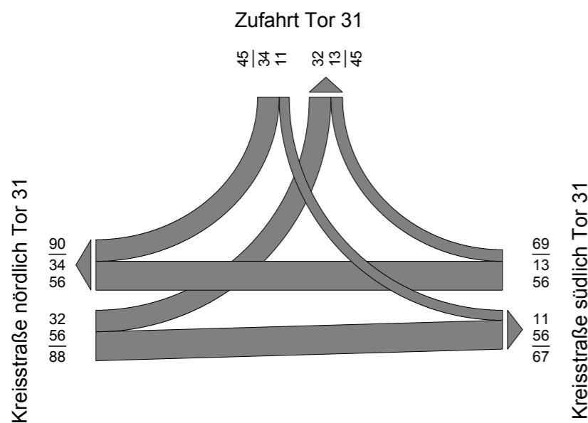
Knotenströme Mittlere Nachtbelastung (22:00 Uhr - 6:00 Uhr) in Kfz/Std.
